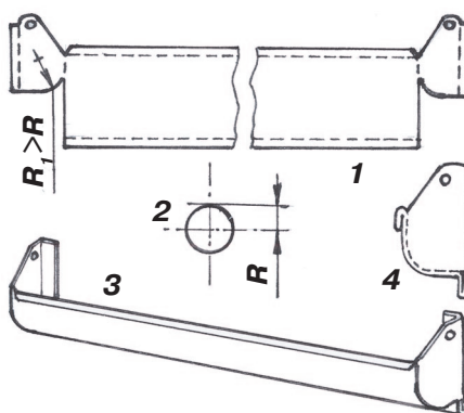
Рис. 3. Конструкция лотка:
