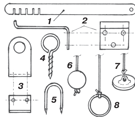
Рис. 4. Общий вид фурнитуры игрового поля: 1 — фиксатор для установки игры, 2 — кронштейн, 3, 4, 5 — варианты «ушек» для тяг, 6, 7, 8 — варианты ручек для управляющих тяг.
